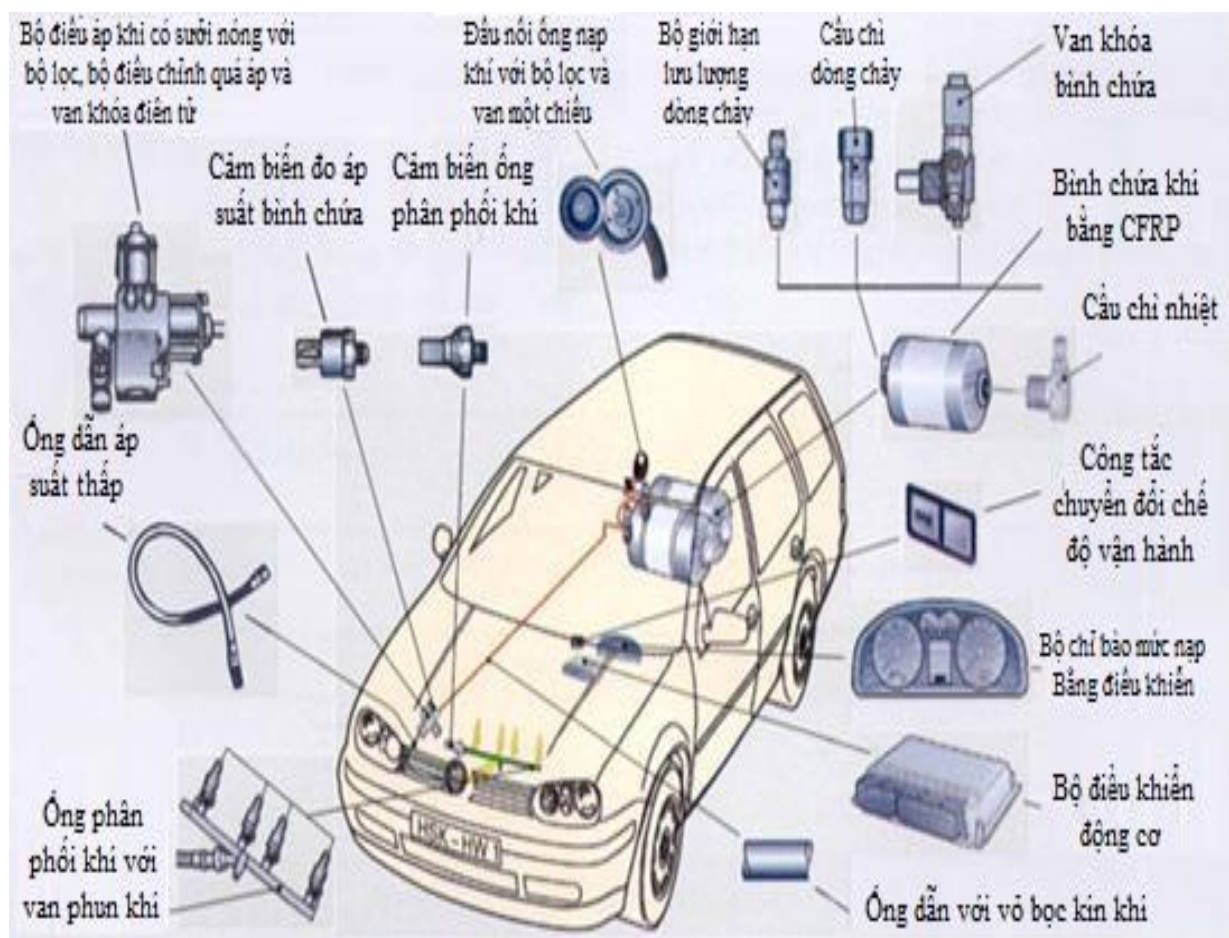
Hình 3.12. Xe chạy khí thiên nhiên
