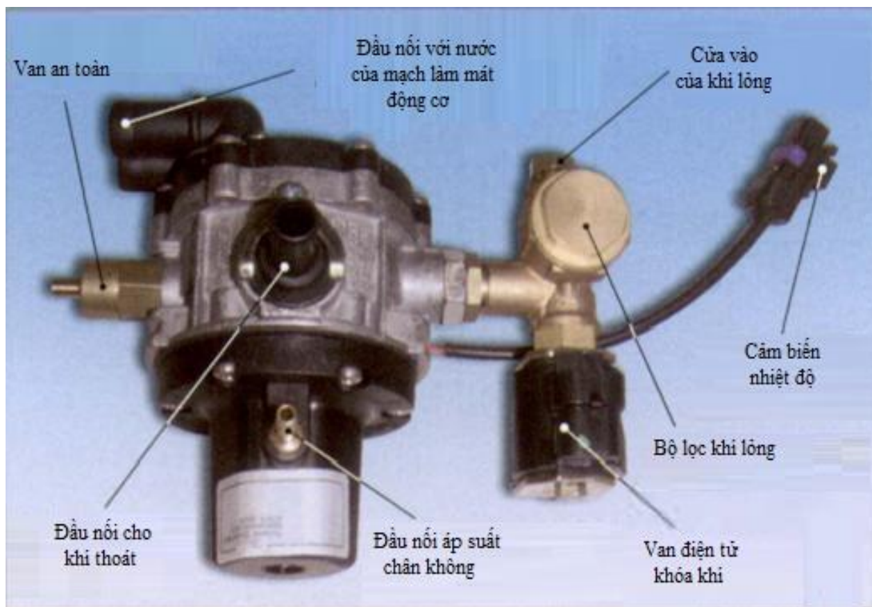
Hình 3. 15. Bộ hoá hơi - điều áp
