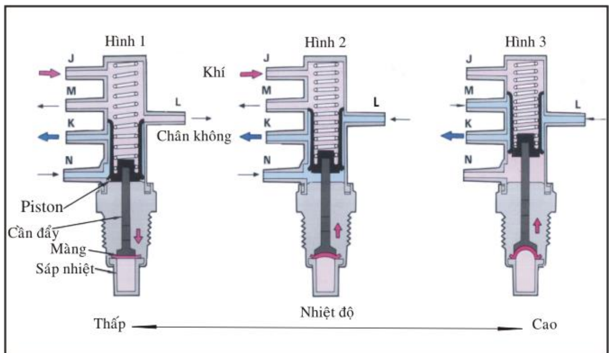
Hình 3.4. Van chân không điều khiển bằng nhiệt
