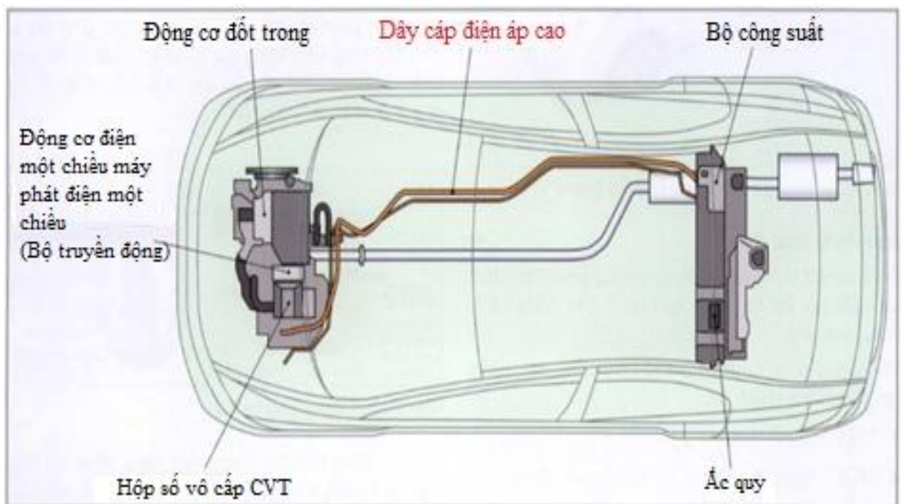
Hình 3. 21. Bố trí trên xe của hệ thống Hybrid song song
