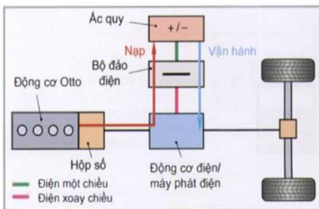
Hình 3. 19. Hệ thống Hybrid song song
