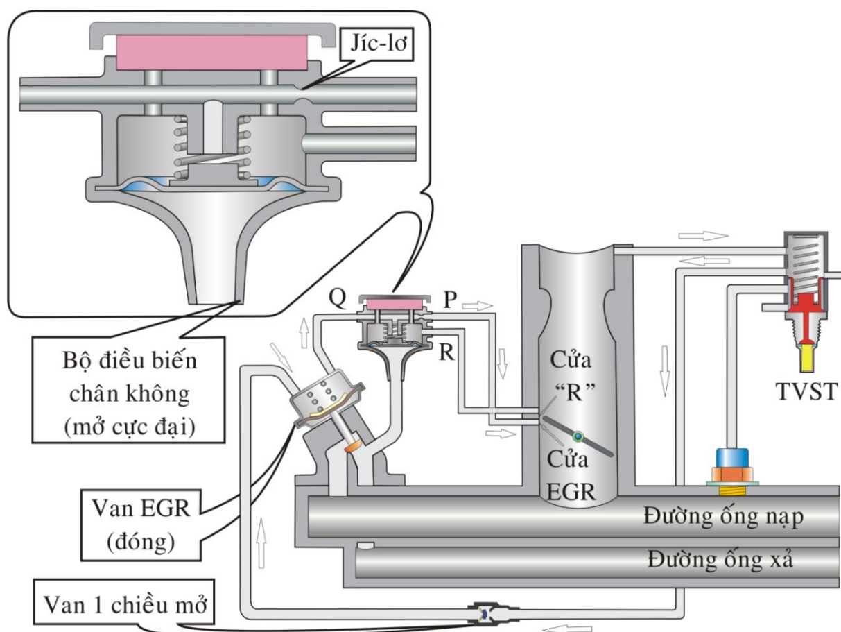
Hình 3. 5. Động cơ lạnh (nhiệt độ nước làm mát dưới 50 °C)
