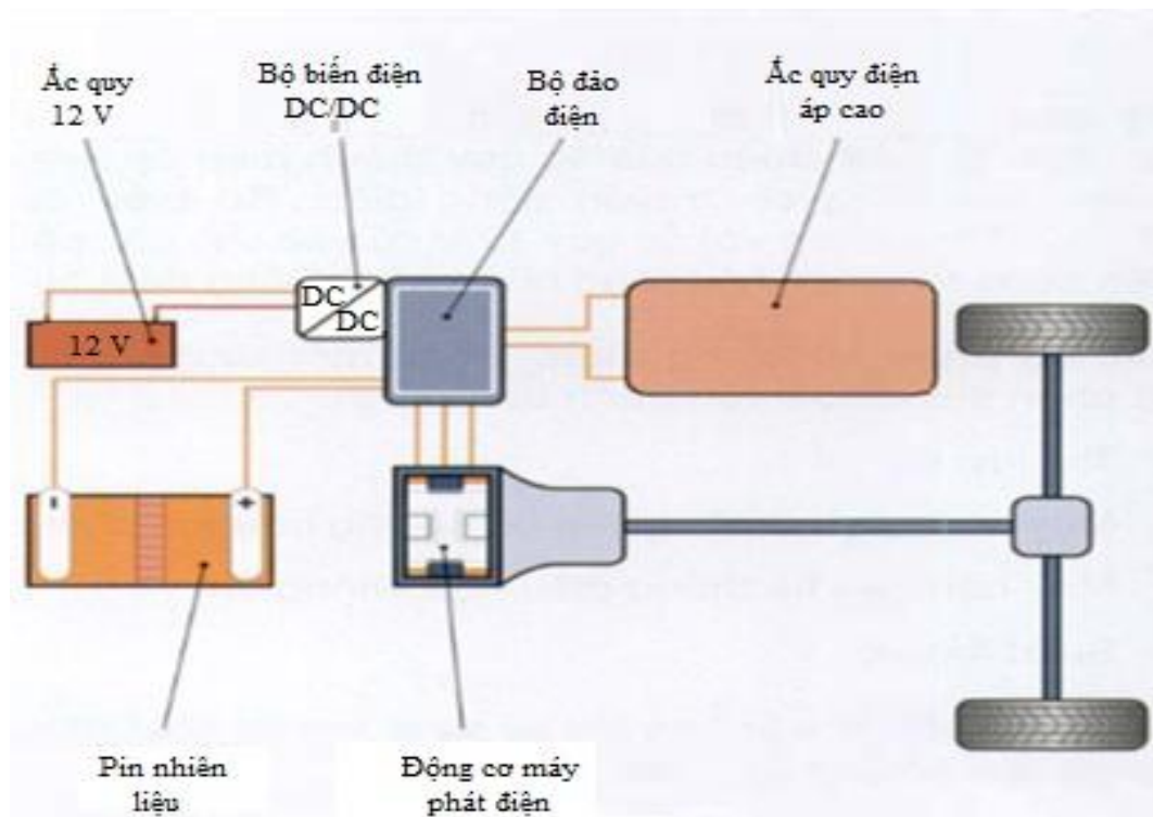
Hình 3. 26. Hệ thống truyền động
