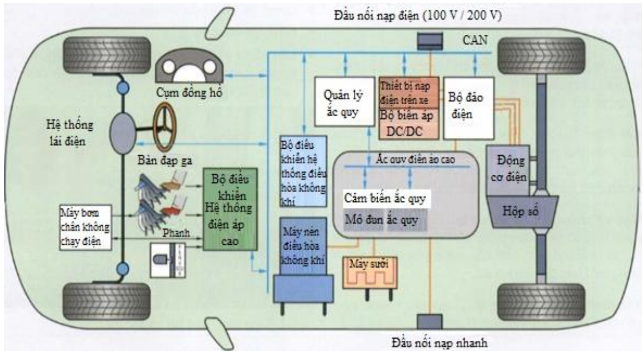
Hình 3.23. Các bộ phận của xe điện
