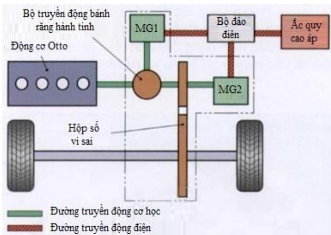
Hình 3.22. Cấu tạo bộ truyền động Hybrid
