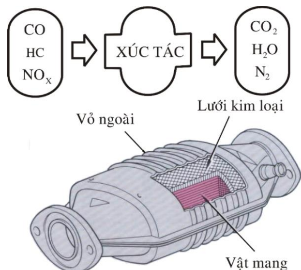
Hình 3. 8. Thiết bị xúc tác
