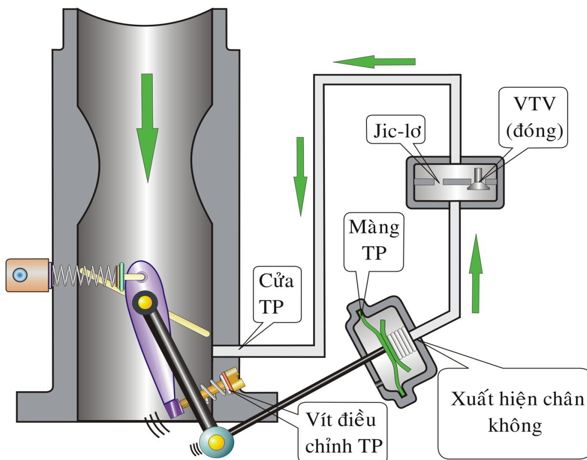
Hình 3.9. Hệ thống điều khiển bướm ga
