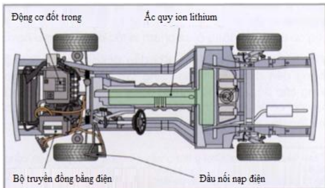
Hình 3. 18. Hệ thống Hybrid nối tiếp
