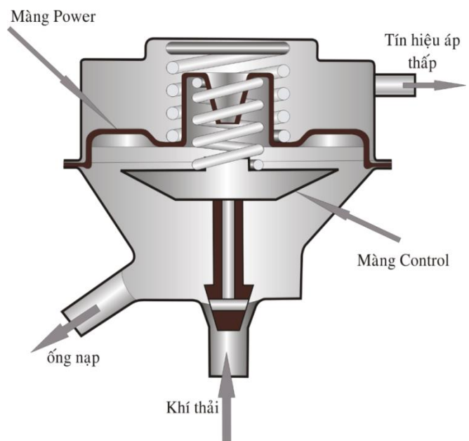
Hình 3.3. Cấu tạo van điều chỉnh áp suất ngược (EGR valve)
