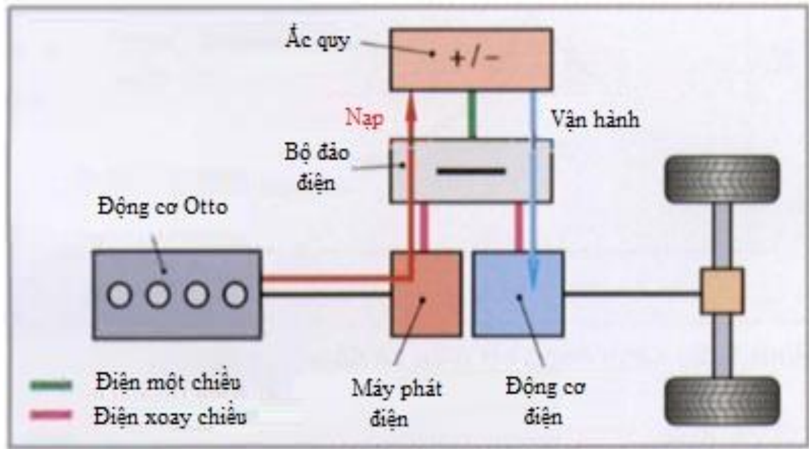
Hình 3. 17. Truyền động Hybrid nối tiếp
