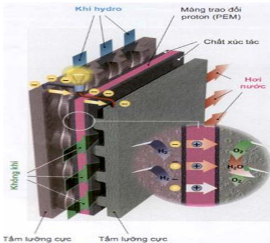
Hình 3.24. Cấu tạo và nguyên lý hoạt động của pin nhiên liệu
