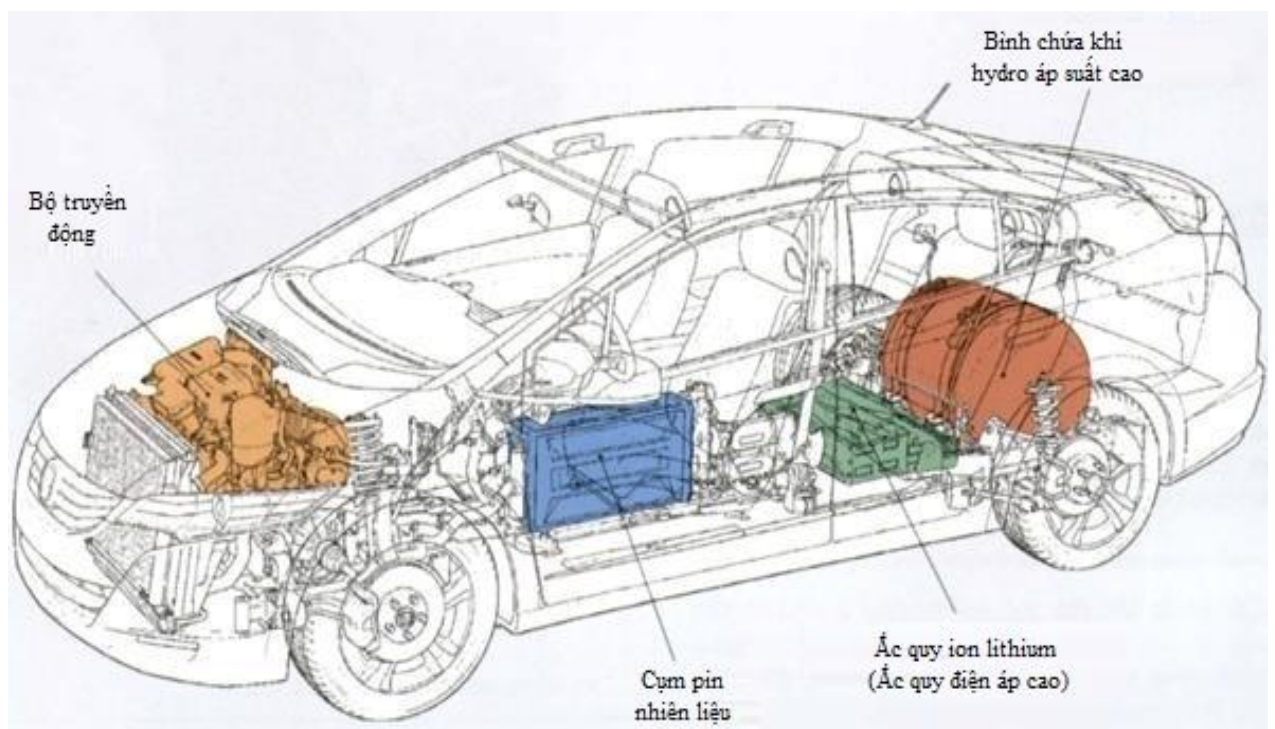
Hình 3. 25. Các bộ phận của pin chạy nhiên liệu
