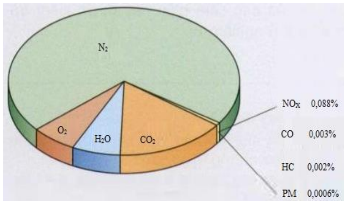
Hình 3. 10. Thành phần khí thải [19]
